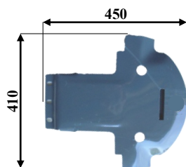
Art: G05 PATTINO senza foro
