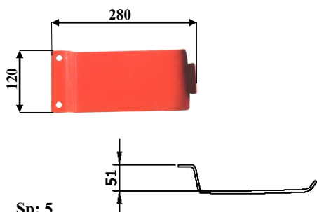
Art: F05 DISCO TRIANGOLARE con pulitori Rif. orig: 90016529 - B2280294
