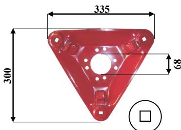
Art: F05 DISCO TRIANGOLARE con pulitori Rif. orig: 90016529 - B2280294
