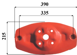
Art: D01 DISCO OVALE Rif. orig: 56808210 - 56812600
