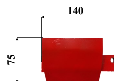
Art: D16 PROTEZIONE ESTERNA Rif. orig: 56808710
