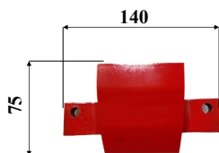
Art: D15 PROTEZIONE CENTRALE Rif. orig: 53808510 AR
